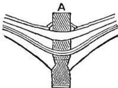
A, Keelson.
